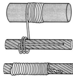
Fig. 59. Wrapping procedure
