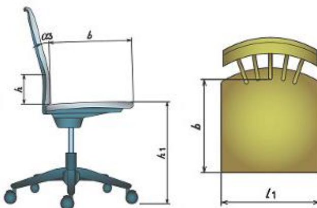
Obr. č. 3.3 Rozměry univerzální židle dle ČSN 91 0620 (NIS)
