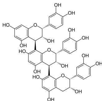
Kondenzovaný tanin (prokyanidin)
