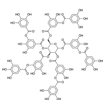
Hydrolyzovatelný tanin (kyselina tříslová)
